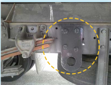
Placas en camión con frenos hidroneumáticos.
